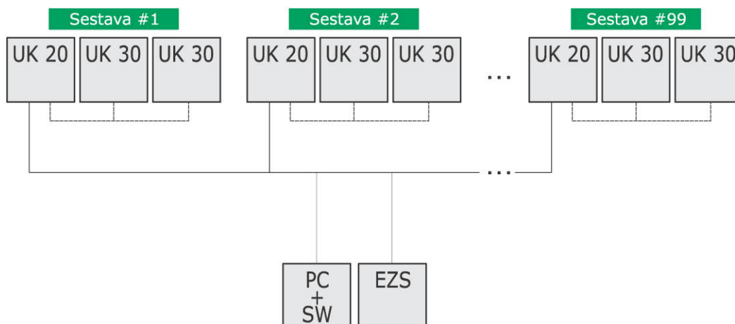
Obr. 5 Blokové schéma propojení sestav úložen klíčů
